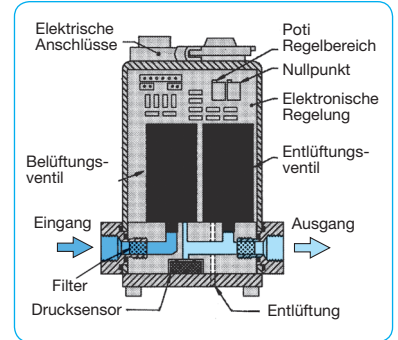
Schnittbild PQ1
